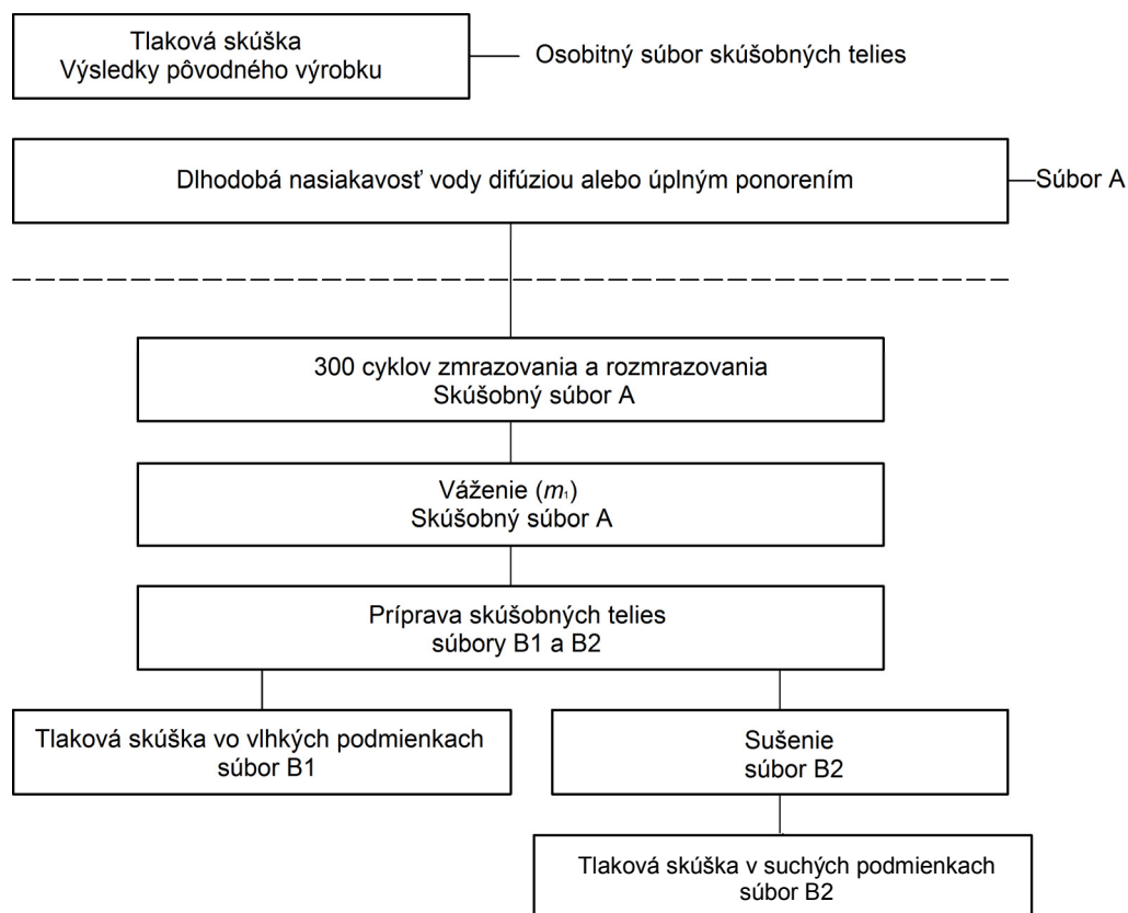
Obrázok 1 – Schéma skúšobného postupu
