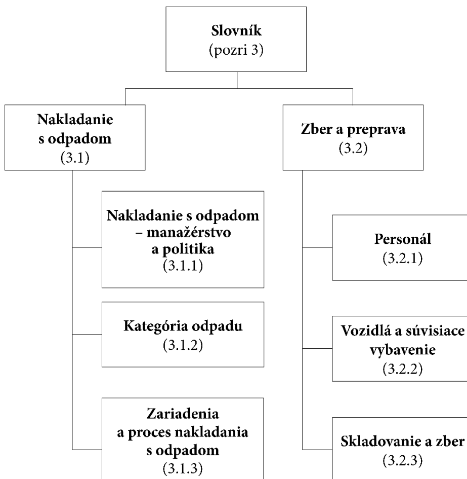
Obrázok 1 – Štruktúra slovníka
